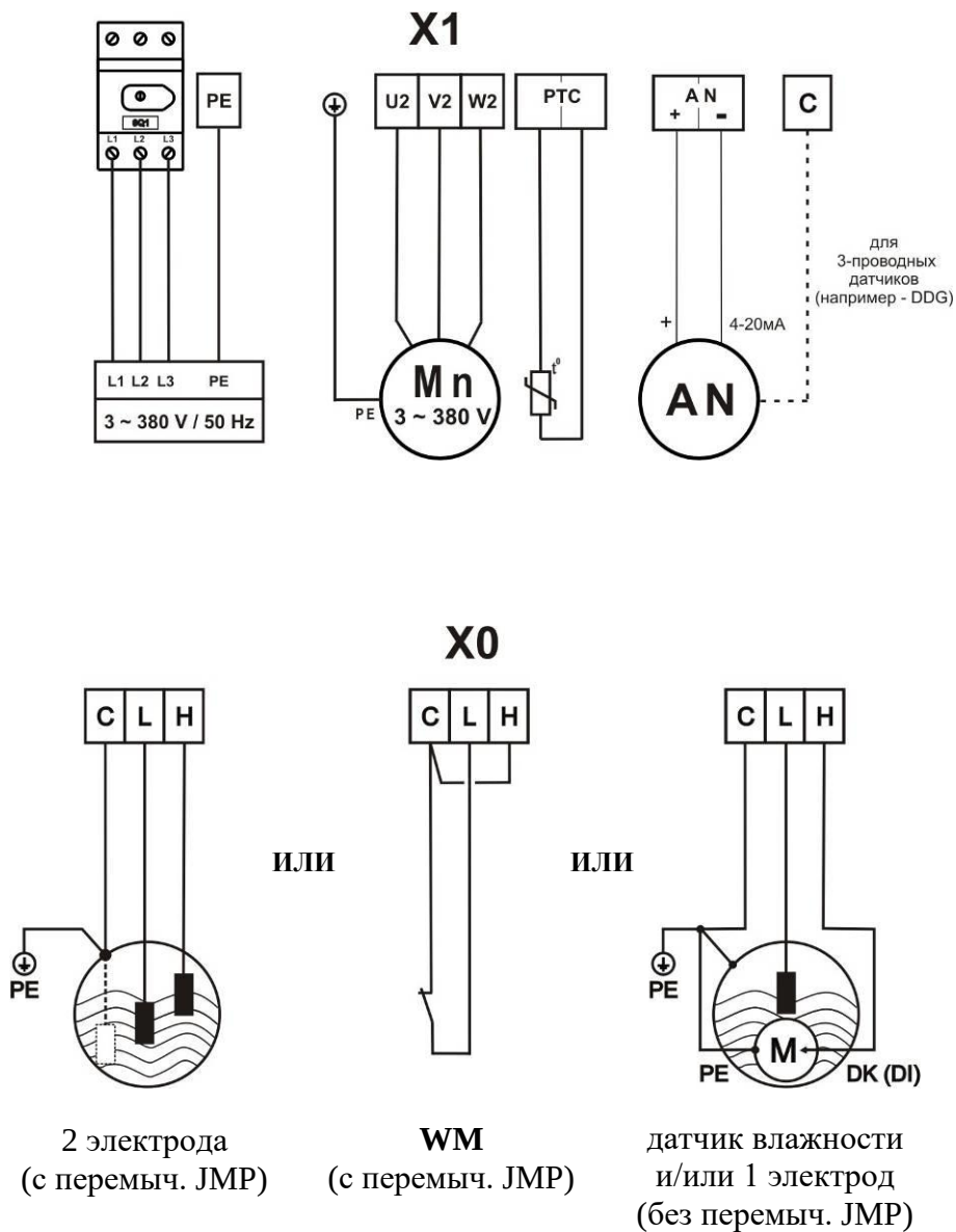
Рис. 3 Подсоединения сетевых контактов и клеммных колодок
